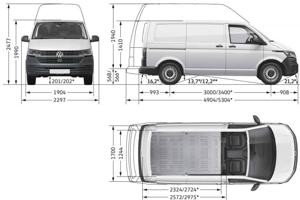
Transporter 6.1 Kastenwagen mit kurzem Radstand und Normaldach/mit langem Radstand und Normaldach/ mit langem Radstand und Hochdach
